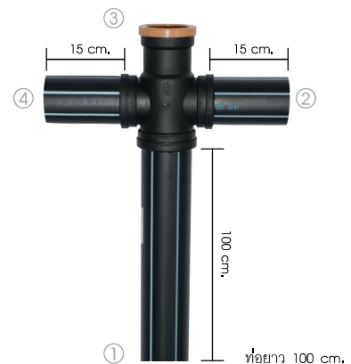
ชุดสี่ทางสำหรับอ่างล้างมือ REDUCING CROSS FOR SINK SET
